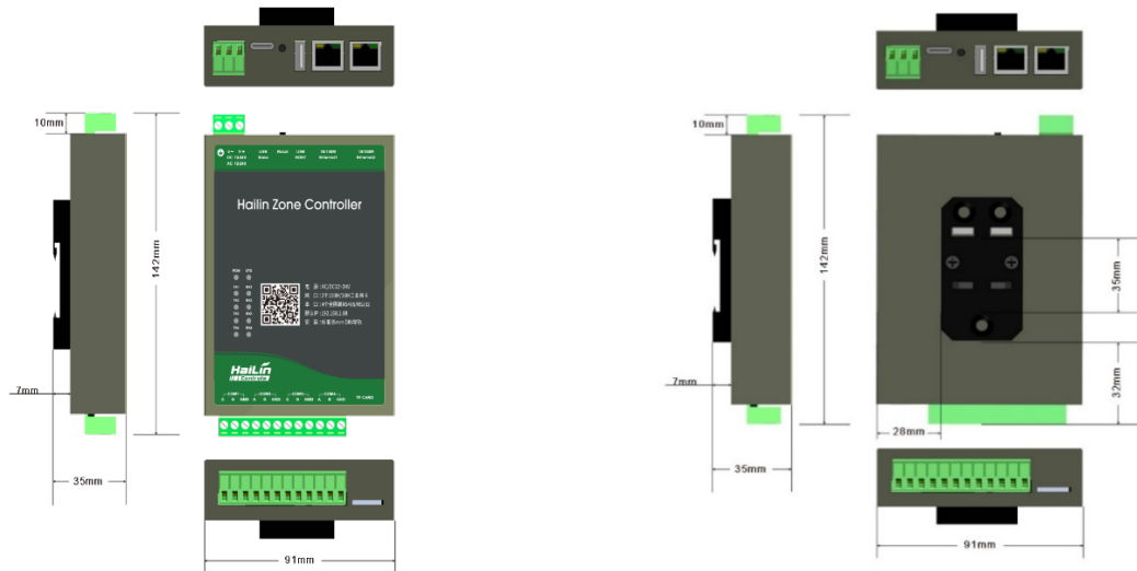
HC-24-2048 尺寸图
