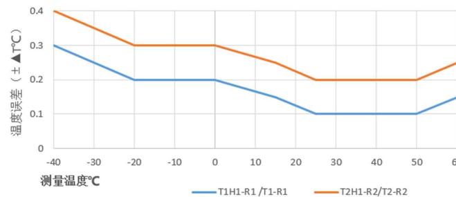
风管道温度精度曲线（电压/电流输出）
