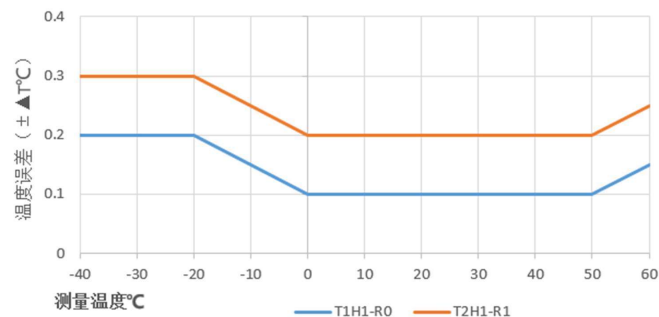
风管道温度精度曲线（RS485输出）
