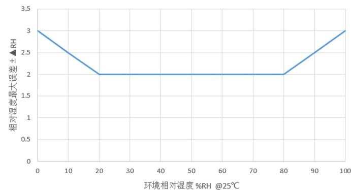
相对湿度精度曲线
