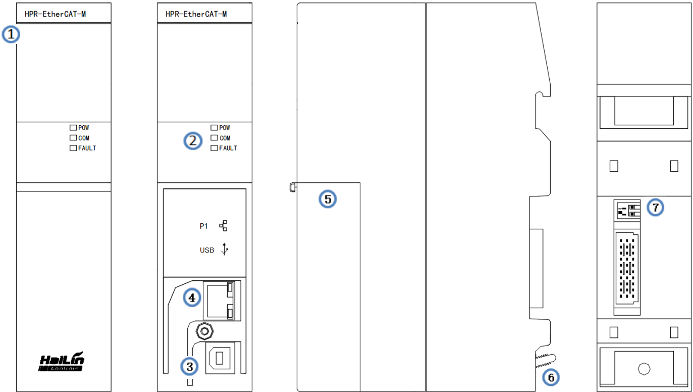
图 1 HPR-EtherCAT-M 结构图
