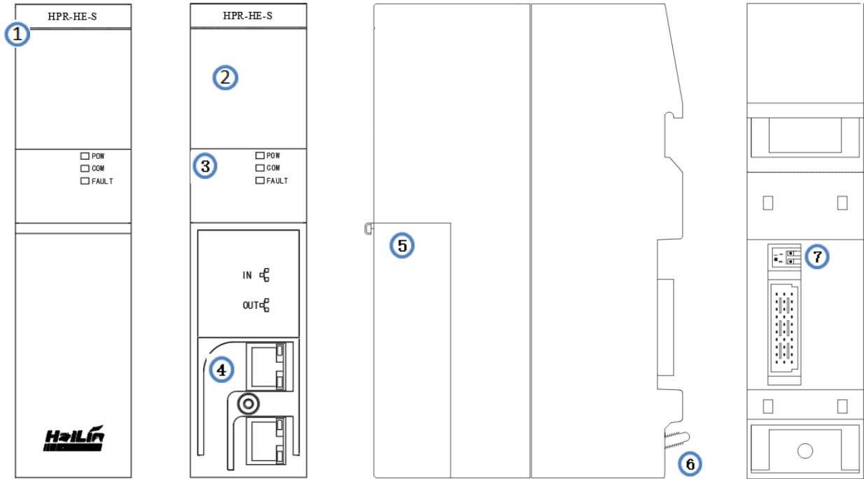
图 1 HPR-HE-S 结构图
