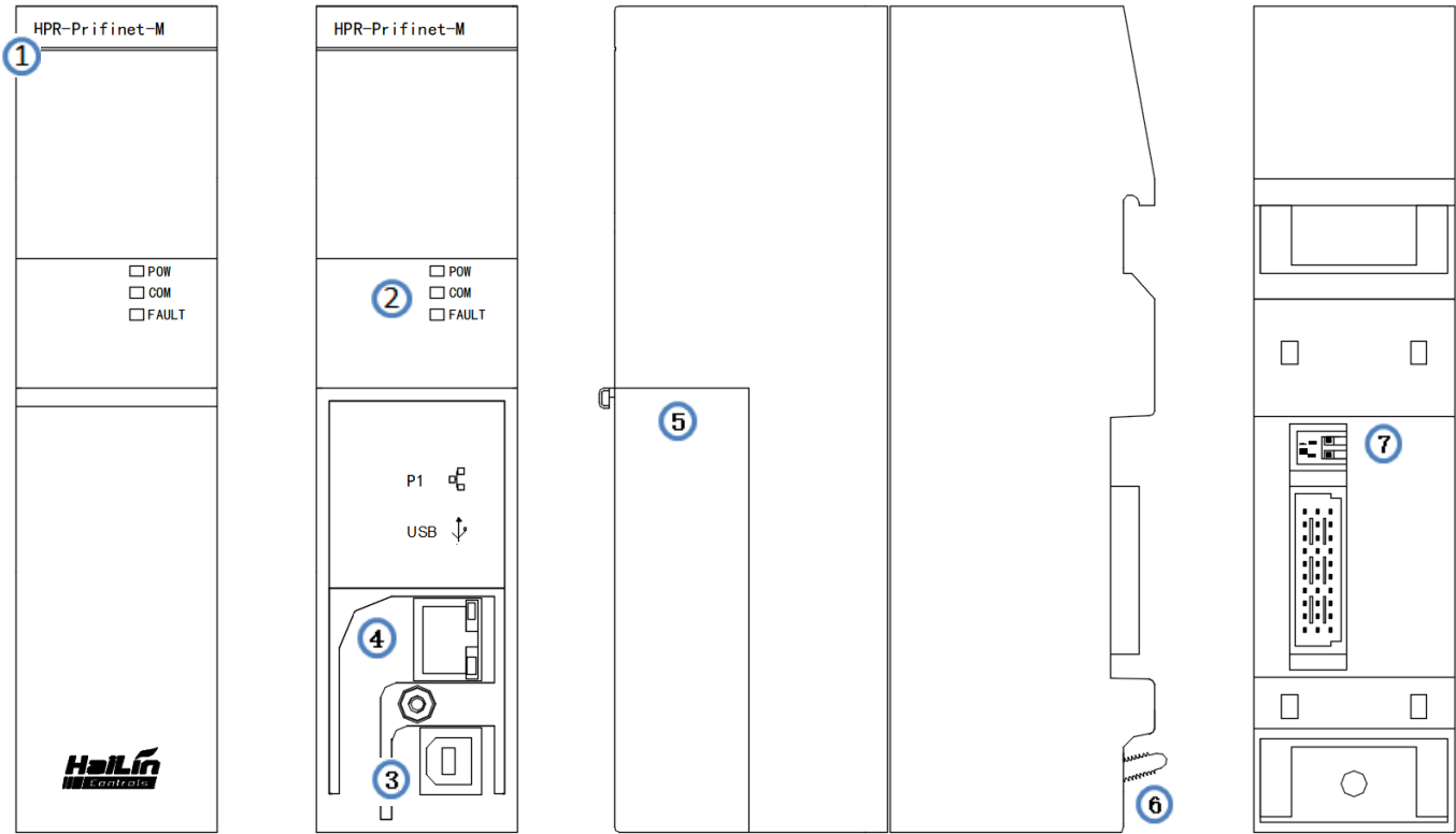
图 1 HPR-Profinet-M 结构图
