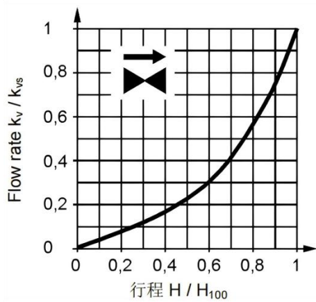
(1) 两通阀流量特性曲线
