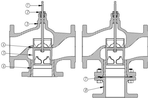
ETF-03（三通阀）
