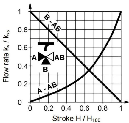
(2) 三通阀流量特性曲线
