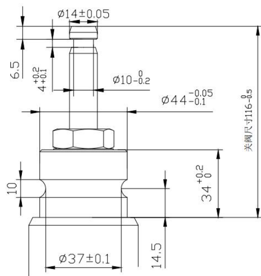
40mm 行程阀体接口尺寸图
