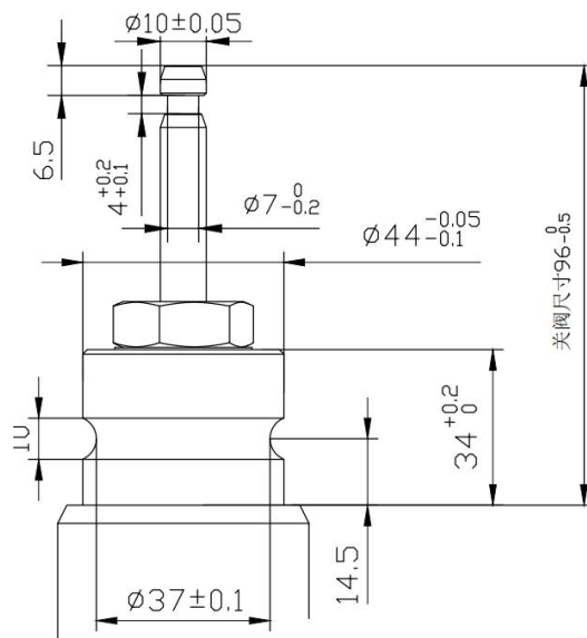
20mm 行程阀体接口尺寸图
