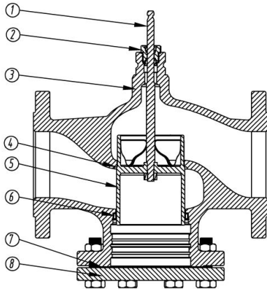
ETF-02（两通阀）
