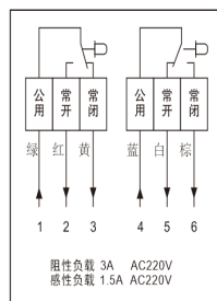
带 2 个位置反馈接线图
