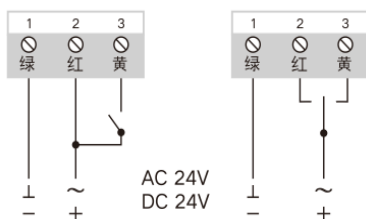
2Nm-40Nm开关型接线图
